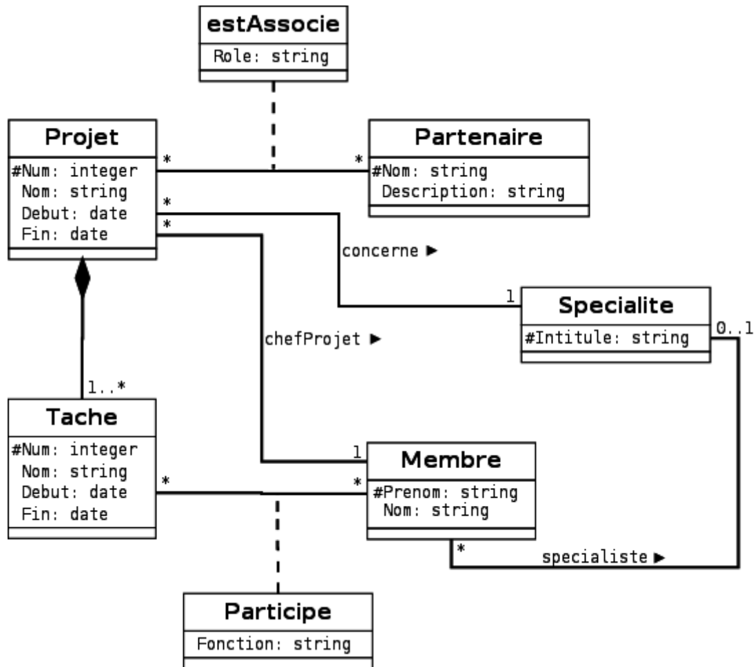
Modèle UML "gestion de projets"
