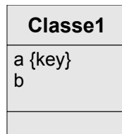
Graphique 3 Attribut
