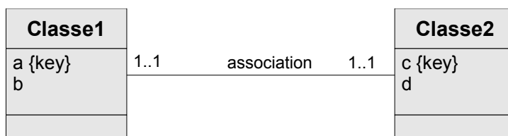
Graphique 21 Association 1:1
