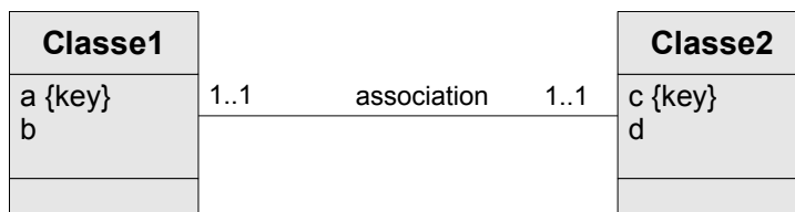
Graphique 10 Association 1:1
