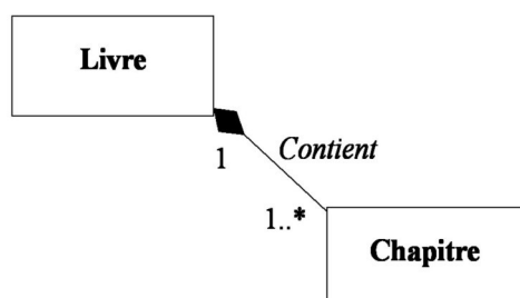
Image 15 Un livre
