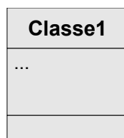
Graphique 2 Classe
