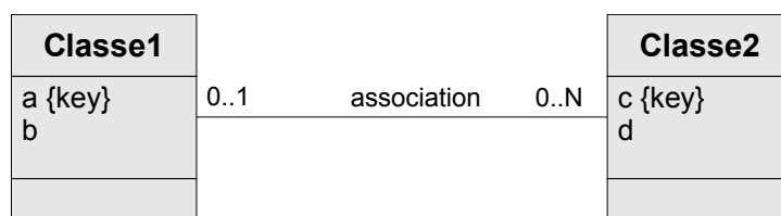
Graphique 8 Association 1:N
