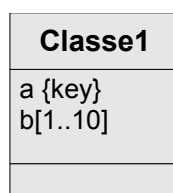
Graphique 5 Attribut multivalué
