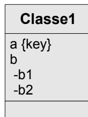
Graphique 4 Attribut composé
