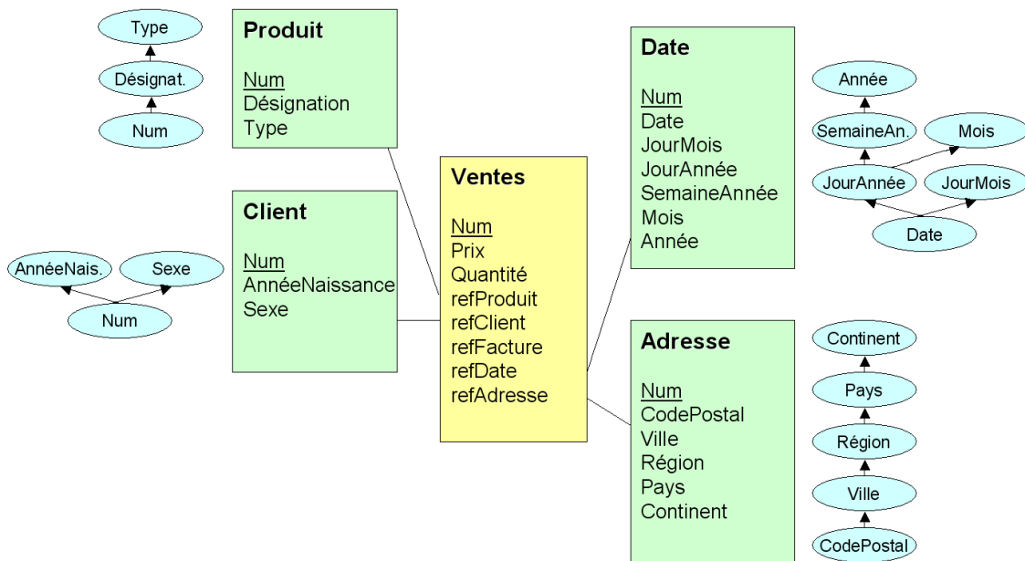
Image 2 Modèle dimensionnel
